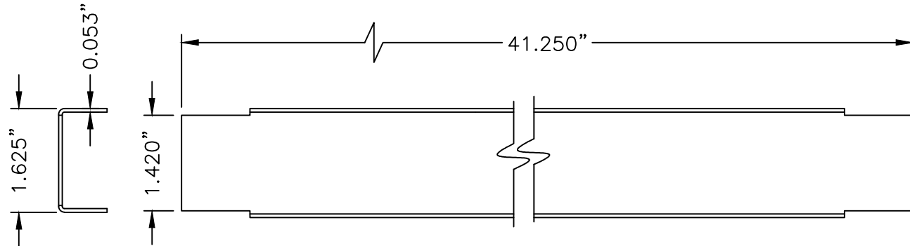
4 DOOR TOP & BOTTOM CLOSER 16GA. (.053) C.R.S.
